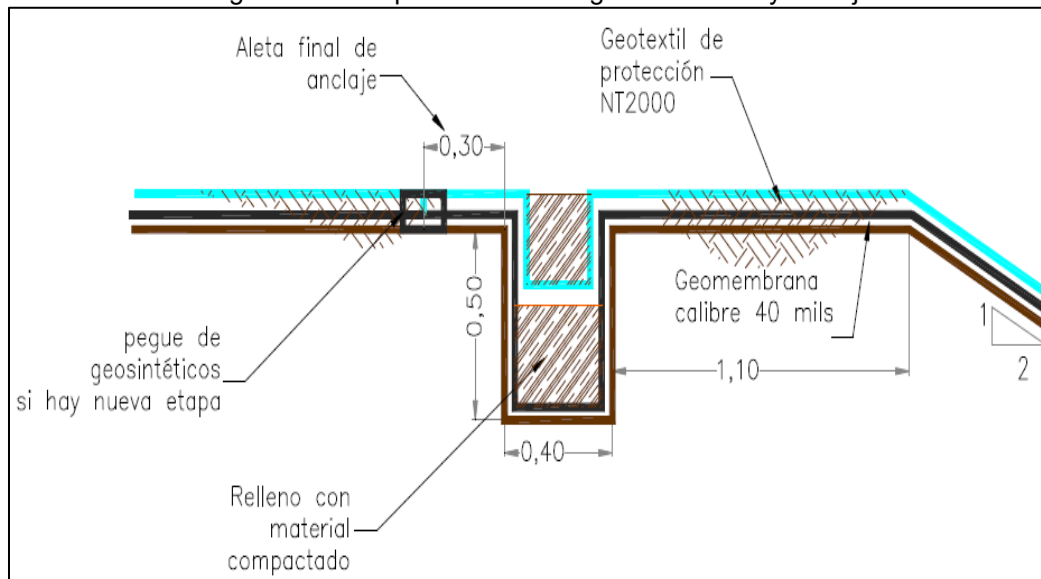
Imagen 21. Perfil protección de la geomembrana y anclaje
