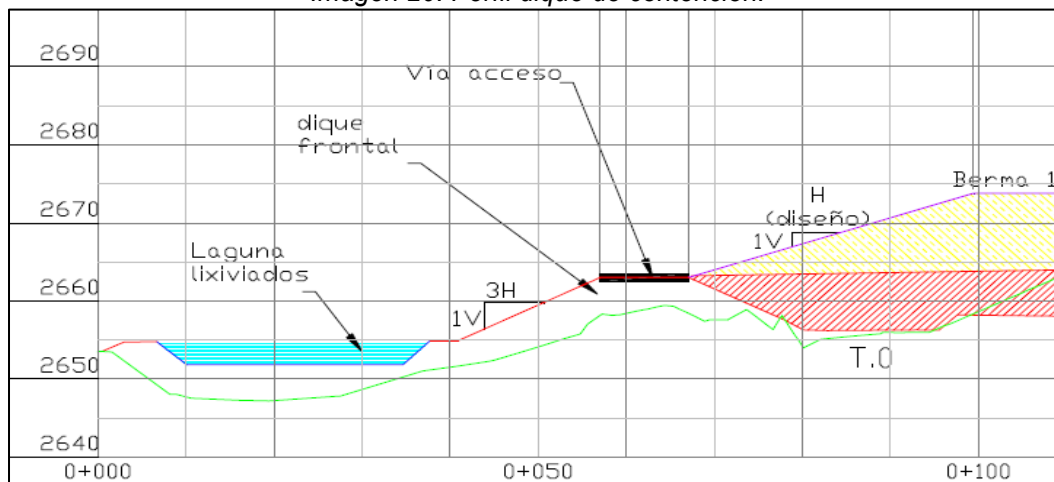
Imagen 20. Perfil dique de contención.
