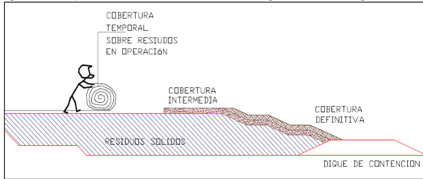
Imagen 10. esquema de cobertura de RSO con geo sintético negro-verde
