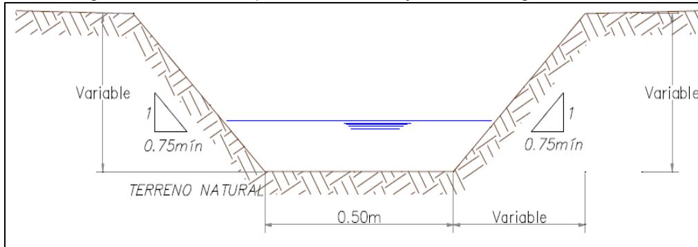
Imagen 14. canales temporales de desvío y control de ingreso de lluvias
