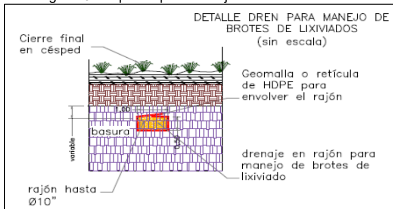
Imagen 23. Esquema para manejo de brotes de lixiviados.
