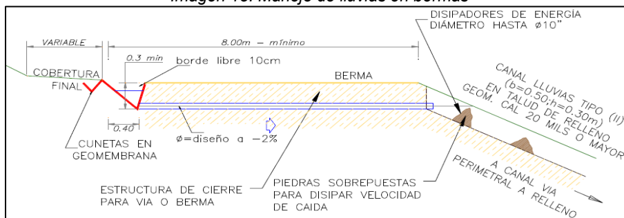
Imagen 15. Manejo de lluvias en bermas
