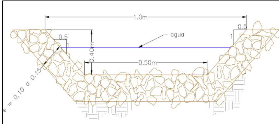
Imagen 16. Ejemplo de canal perimetral en piedra pegada para manejo de aguas lluvia
