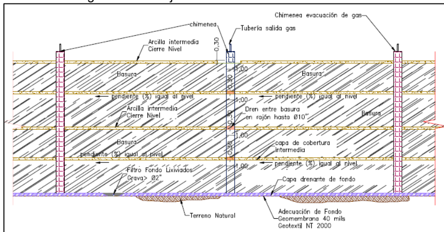
Imagen 22. Drenaje intermedio de la masa de residuos.
