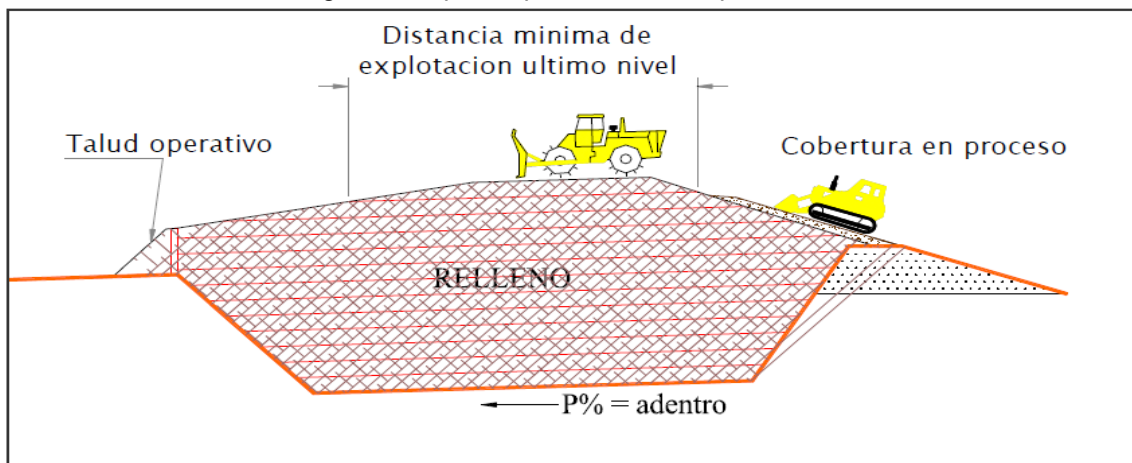
Imagen 9. Esquema proceso de Compactación
