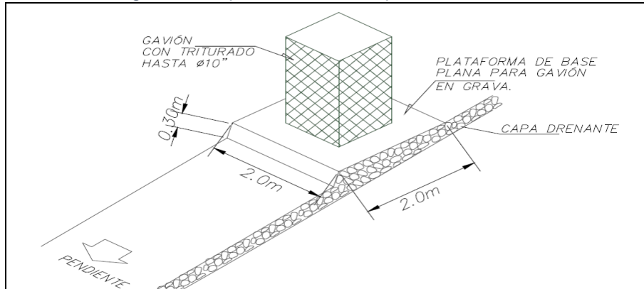
Imagen 19. Esquema Ubicación óptima de Chimeneas
